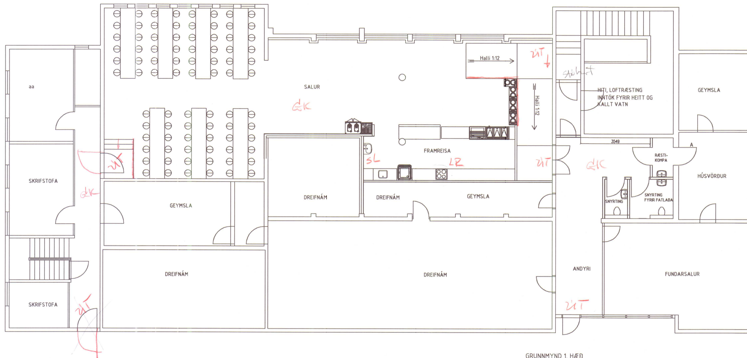
GRUNNMYND 1. HÆÐ MKV 1:100
